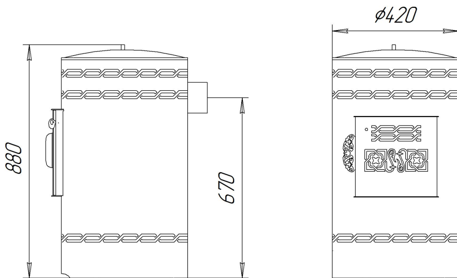
Рисунок 4. Общий вид печи с нанесенными основными размерами
